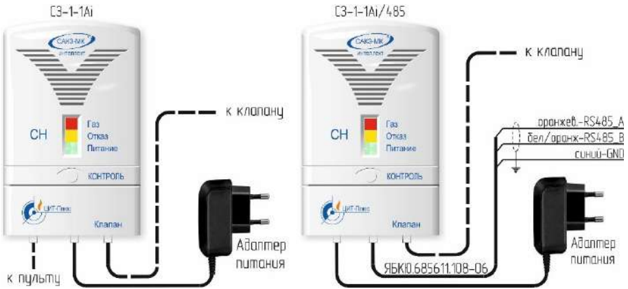
Рисунок В.1 – Типовые схемы включения
